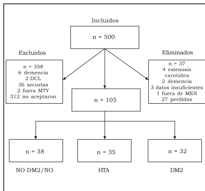
Figura 1. Algoritmo.
